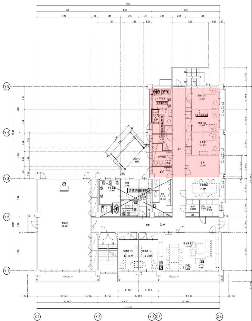
2 階平面図 1/100
