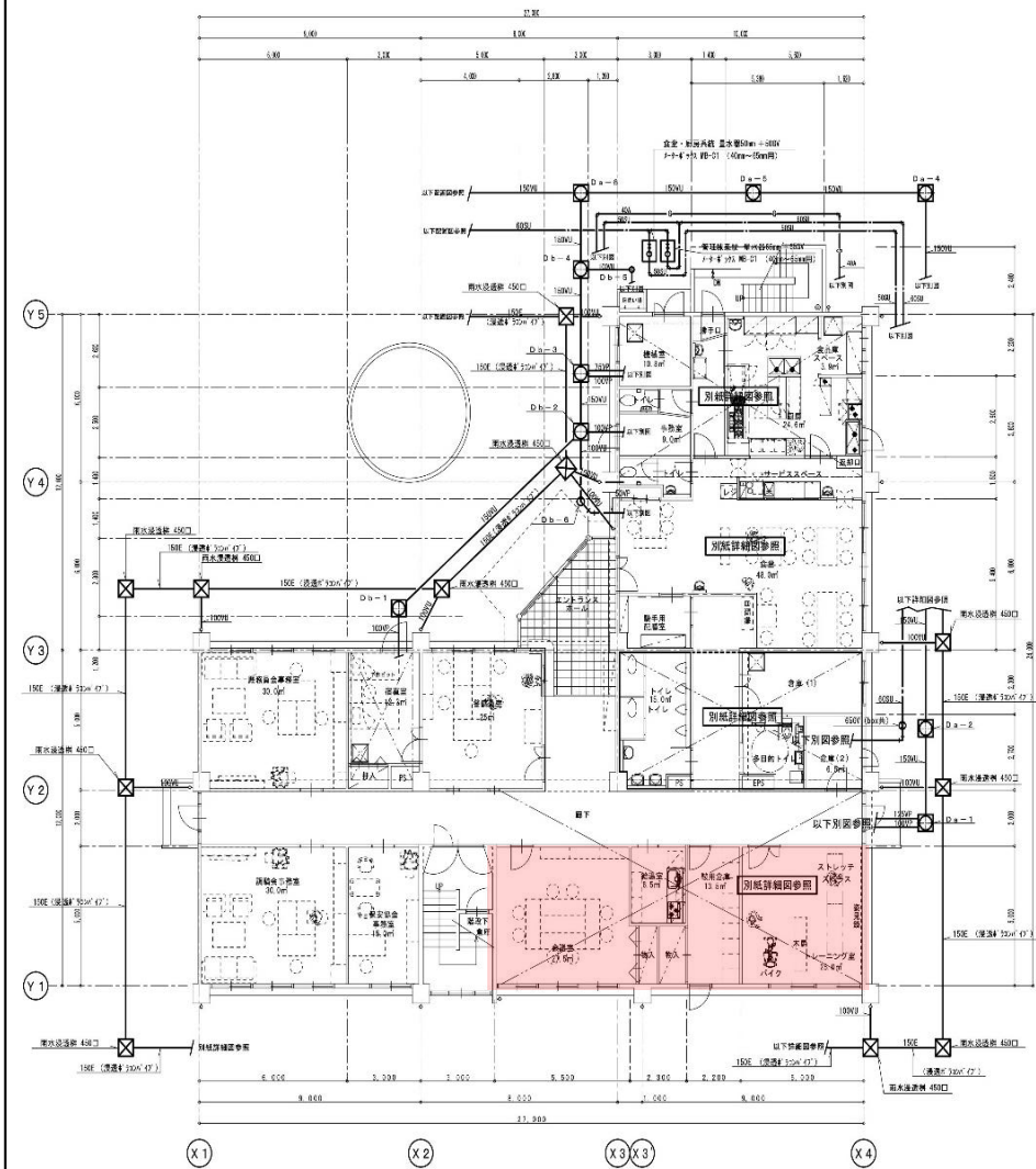
1 階平面図 1/100
