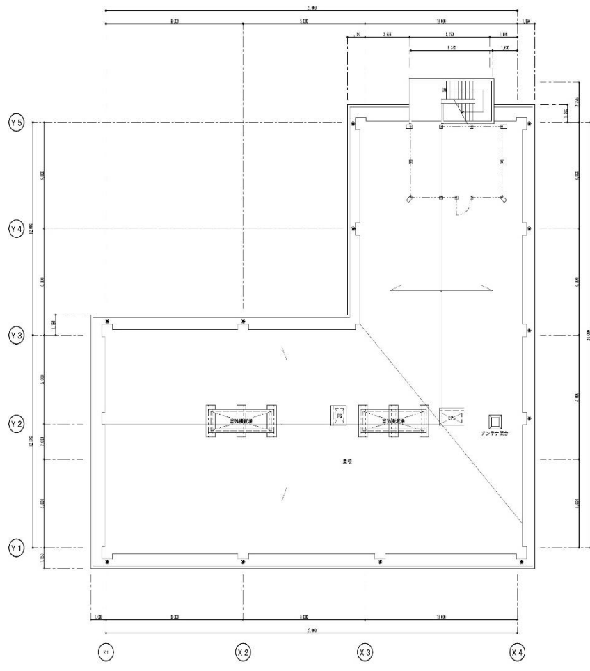
4階平面図 1/100
